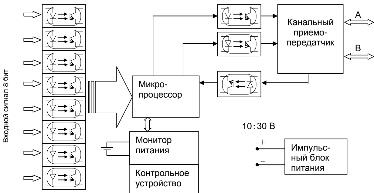
Рисунок 2 – Структурная схема MC1202I
