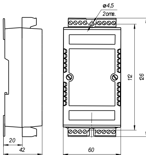
Рисунок 1 – Габаритные и присоединительные размеры МС.
