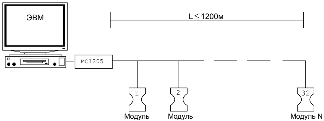
Рисунок 5 – Схема подключения нескольких устройств MC.
